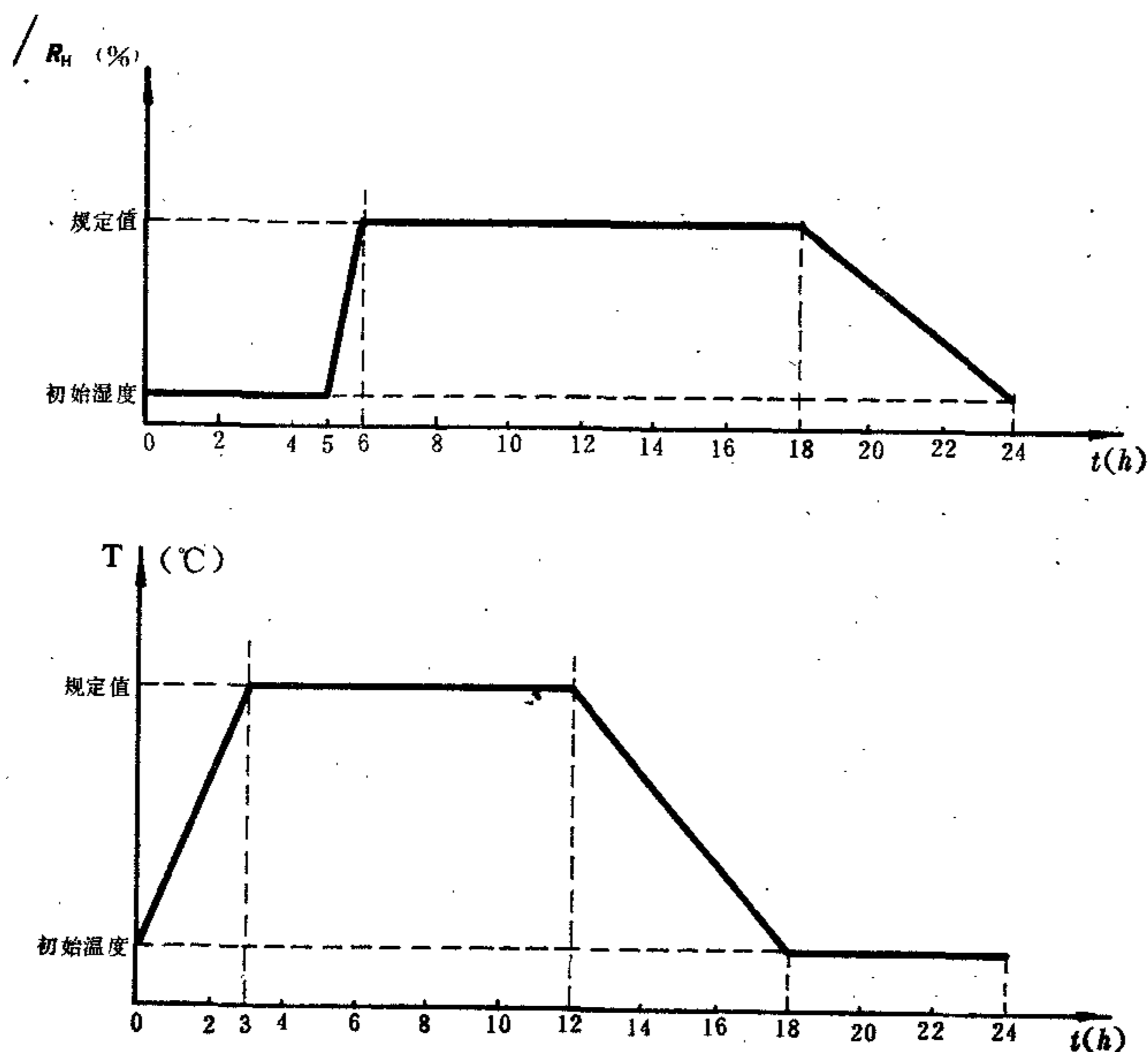
交变湿热试验控制图
